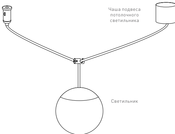
Рис. 1. Установка подвеса
