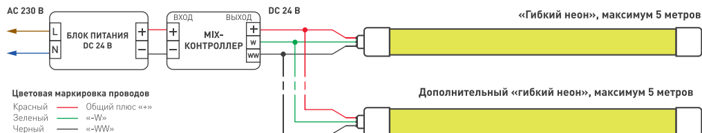
Схема 2. Подключение «гибкого неона» с использованием MIX-контроллера с возможностью изменения цветовой температуры и яркости
