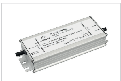
024268 Блок питания ARPV-UH24100-PFC (24V, 4.0A, 96W)
